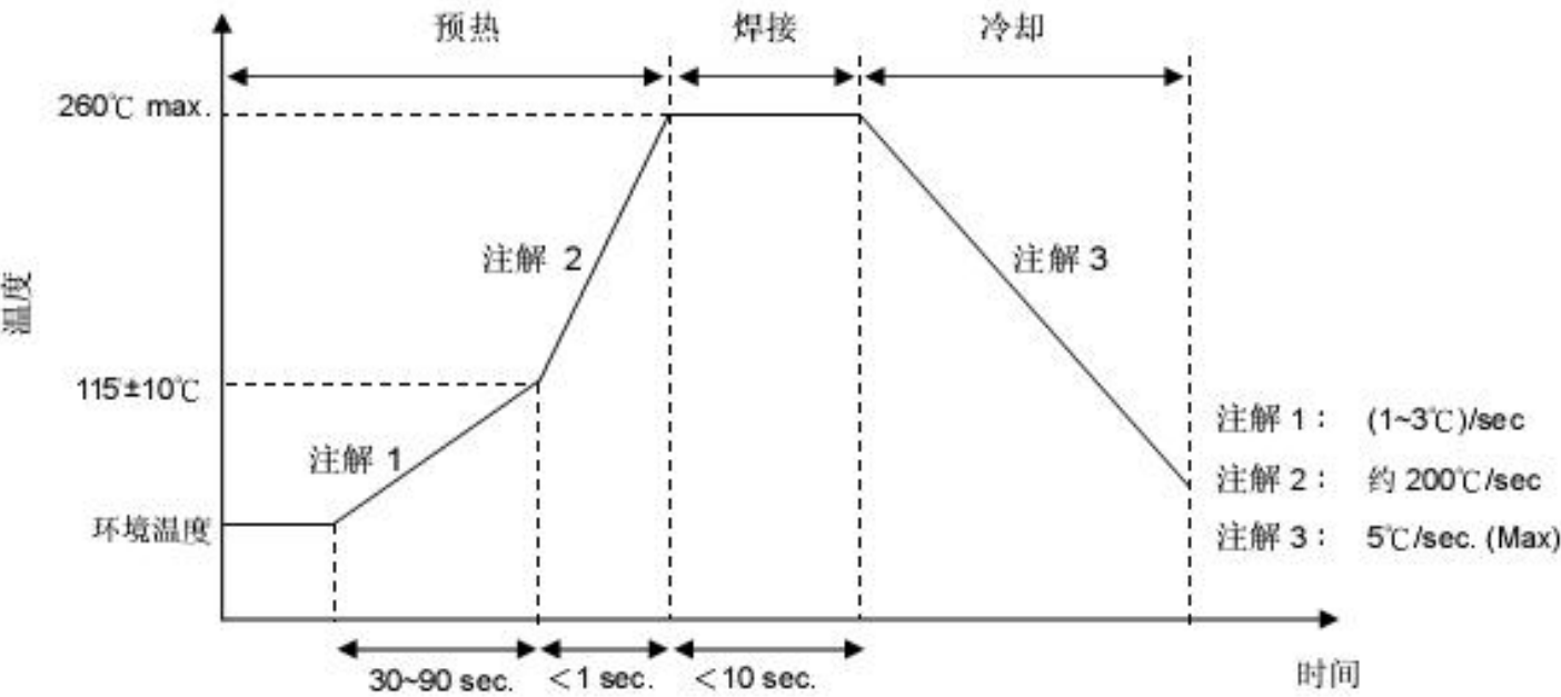
波峰焊曲线
