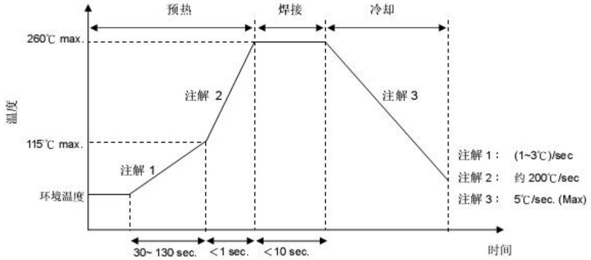
波峰焊曲线
