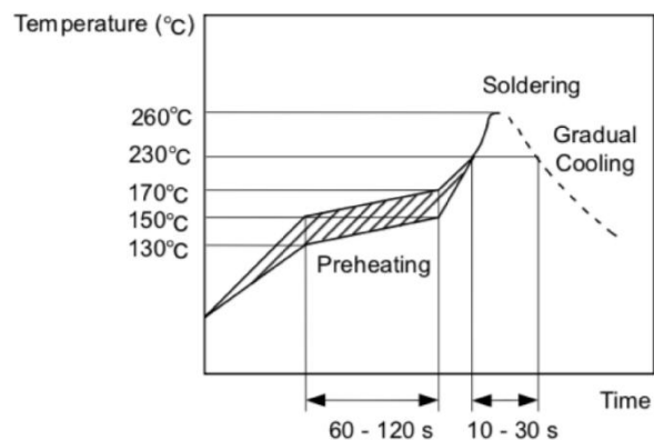
■ 无铅回流焊接曲线
