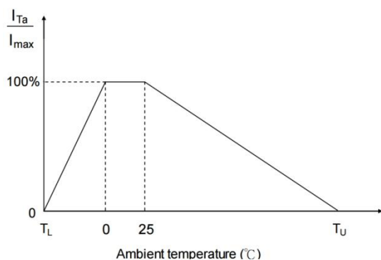
■ 最大电流降额曲线图
